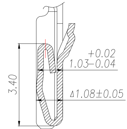
SECTION D-D 2:1
