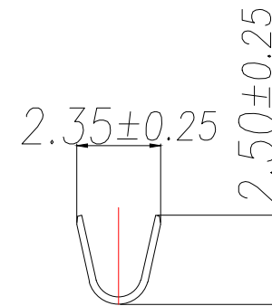
SEC:A-A
