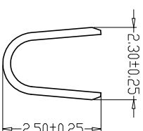
SEC:A-A
